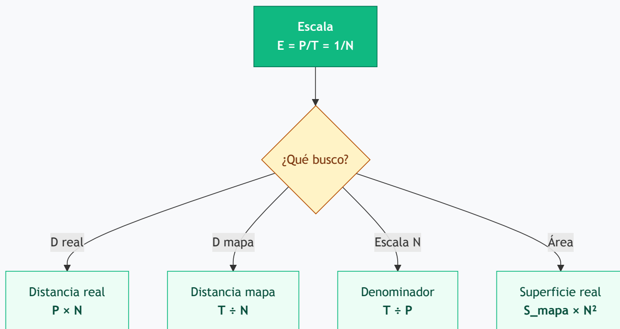
Figura 1 — Decisión de cálculo con escala 1:N (P = distancia en plano, T = distancia en terreno)
